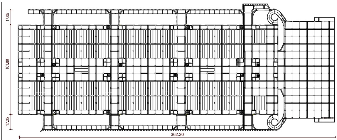
Ολυμπιακό Κέντρο Ραδιοτηλεόρασης: Ξυλότυπος οροφής υπογείου
